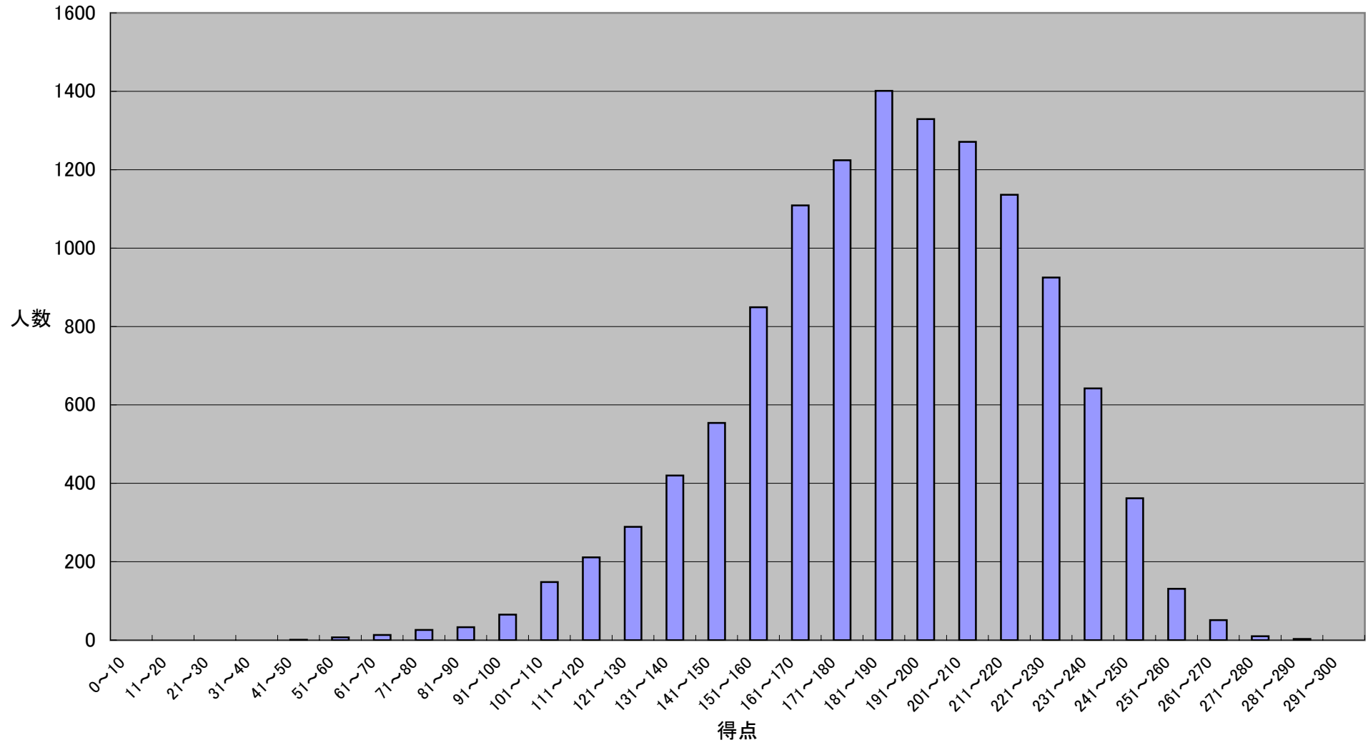
統一適性試験 総合得点 度数分布
